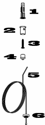
Abb. 2: Stahlseilaufhängung
