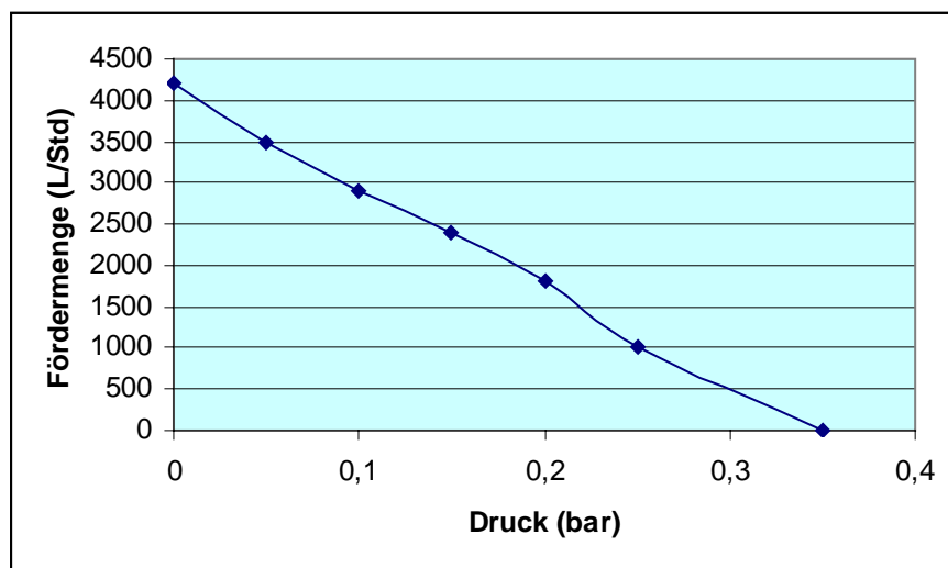
Pumpenkennlinie der Mistral 4000
